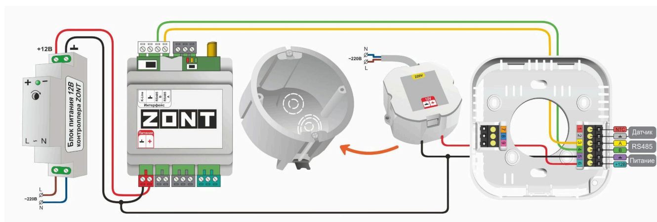
питание Термостата от отдельного блока питания
