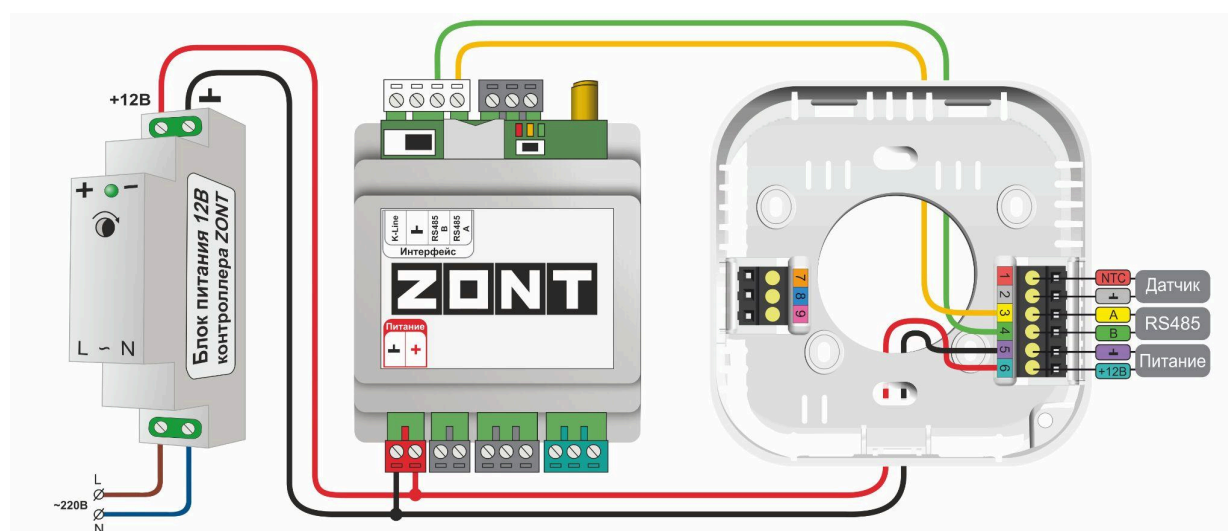
питание Термостата от устройства ZONT
